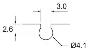
※ C 型溝槽尺寸圖
