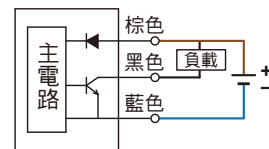
(NPN 輸出)
