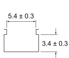
※ T 型溝槽尺寸圖
