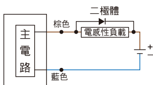
二線式類型
