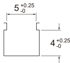
※ T 型溝槽尺寸圖
