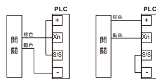
PLC輸入模組 (NPN) PLC輸入模組 (PNP)
