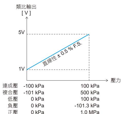
KP10□ - 01 - □ - □
