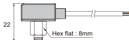
KP10□ - 01 - M5
