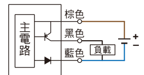
(PNP 輸出)
