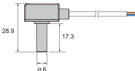
KP10□ - 01 - R6
