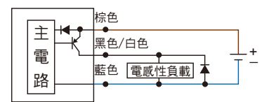
PNP類型
