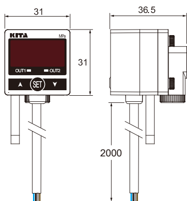
KP25 □ - □ - □
