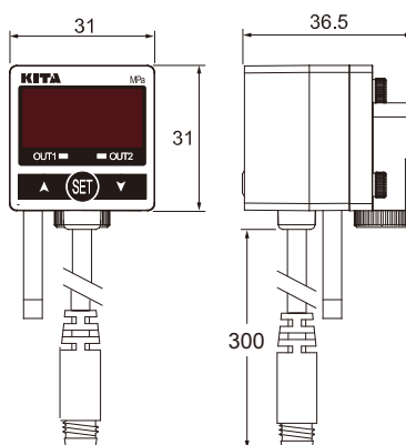
KP25 □ - □ - □ - QD
