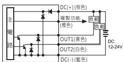
Kp45S-02-□ 2 NPN+複製功能
