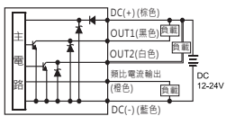
KP45S-011-□ 2 NPN+類比電流輸出 (4~20mA)
