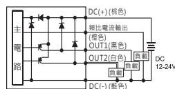
KP45S-031-□ 2 PNP+類比電流輸出 (4~20mA)
