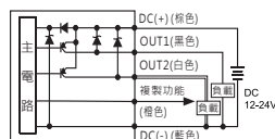
KP45S-04-□ 2 PNP+複製功能
